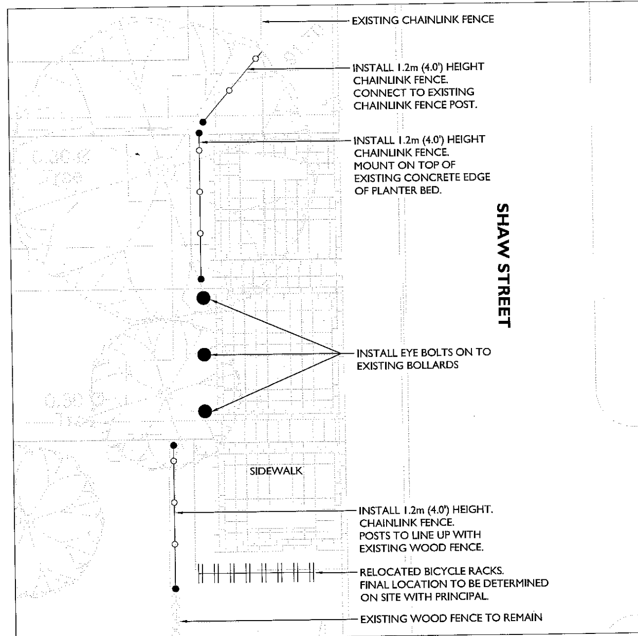
AREA 'B' 1:100
