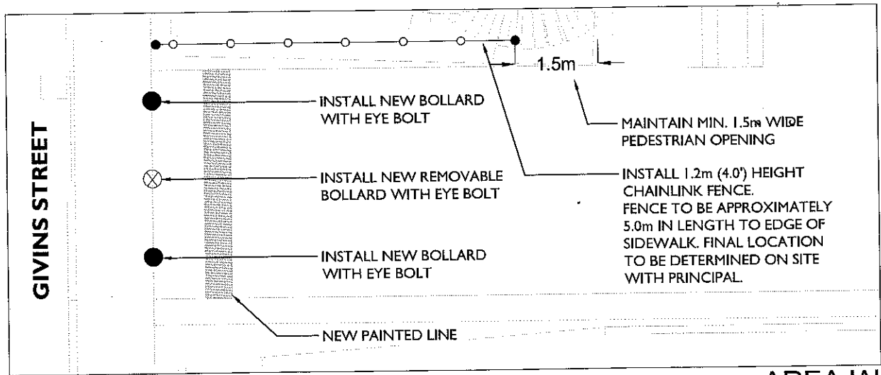
AREA 'A' 1:100
